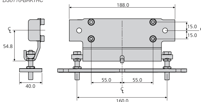
DS0116-BRKTRC
